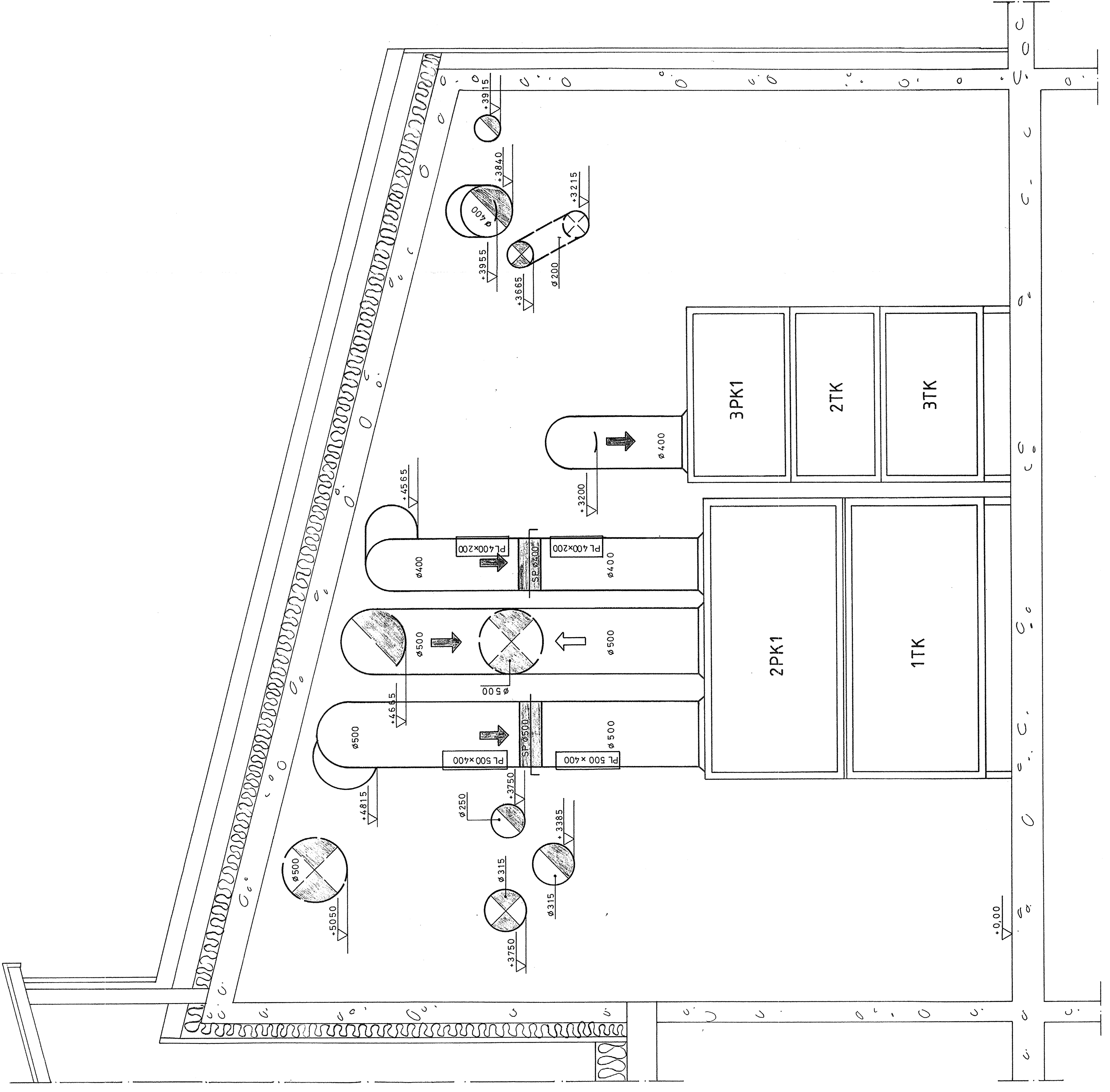
LEIKKAUS 5-5 / 1:20
