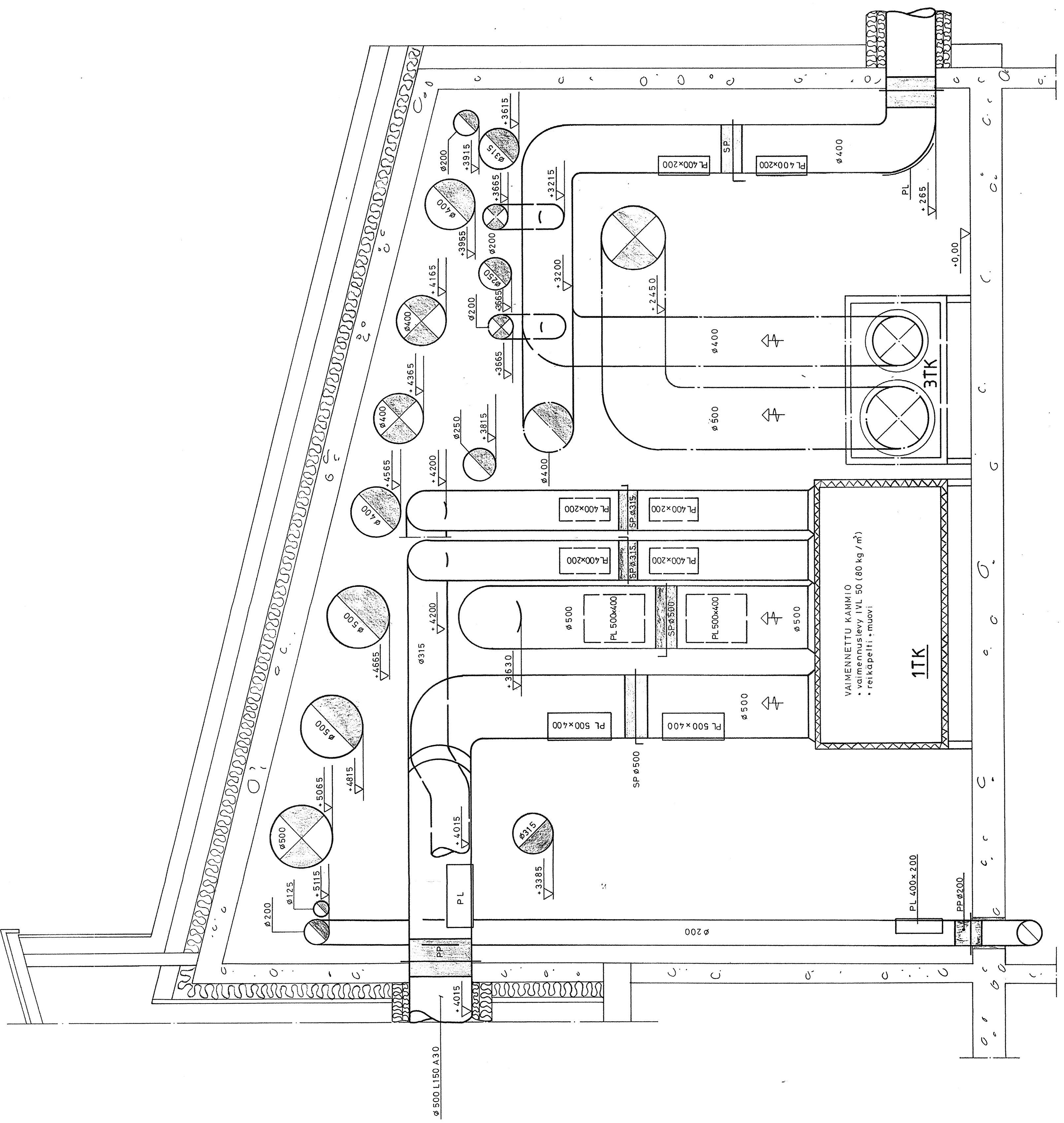
LEIKKAUS 4-4 / 1:20
